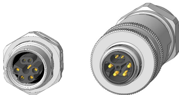
Bild 8: Hybrider M12 SPE Steckverbinder nach IEC 63171-7 (Quelle: TE)
